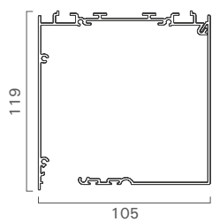
CASSONETTO - C104
