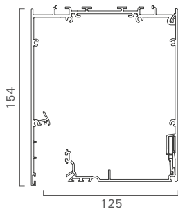
CASSONETTO - C124
