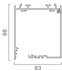
CASSONETTO - C91
