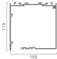
CASSONETTO - C104
