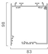
CASSONETTO - C91
