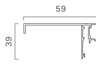
opzioni profilo chiusura incasso optional cover for encasement SUPPLEMENTO - SUPPLEMENT
