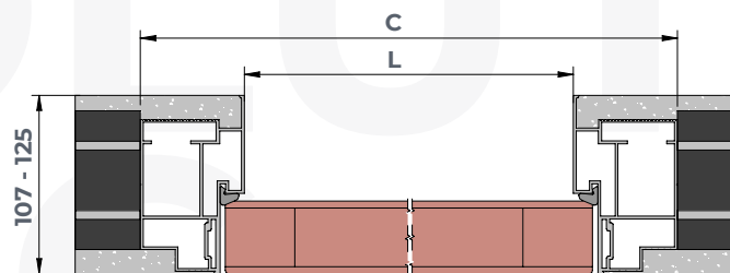
APERTURA A TIRARE
