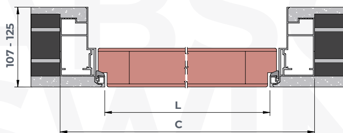
APERTURA A SPINGERE
